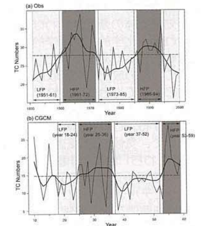
図4. 台風の発生数の数十年変動。(a)観測結果、(b)CGCM結果
