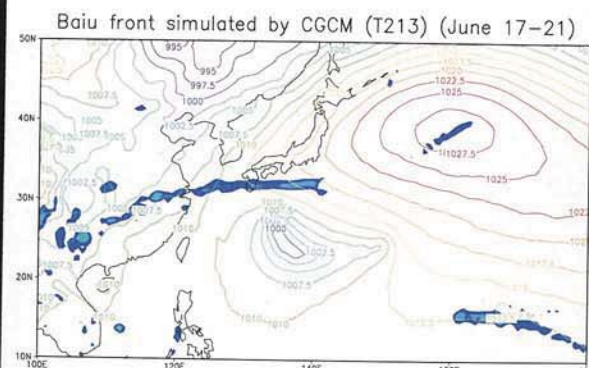
図2. CGCMで再現された梅雨前線
